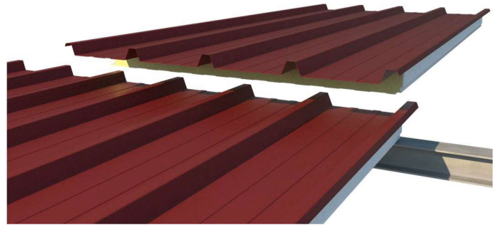
2. Sobald die erste Paneelereihe fertiggestellt ist, das erste Paneele überlappen.
