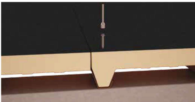
Das Bohrloch muss bis zur darunter befindlichen Sicke reichen.
